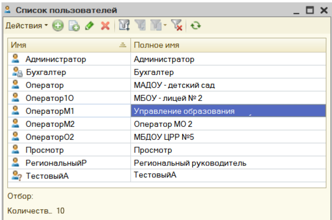
Рисунок 5 – Список пользователей
