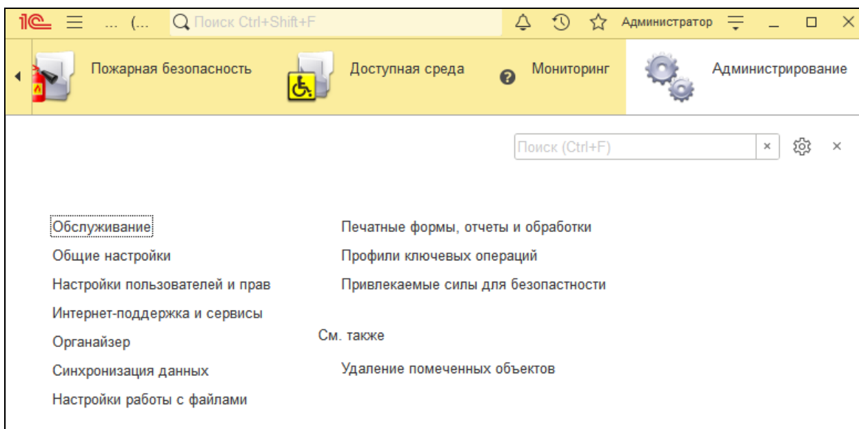
Рисунок 15 – Подсистема «Администрирование»
