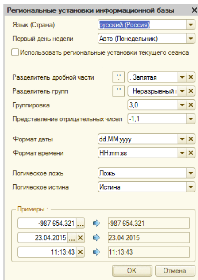
Рисунок 12 – Региональные установки
